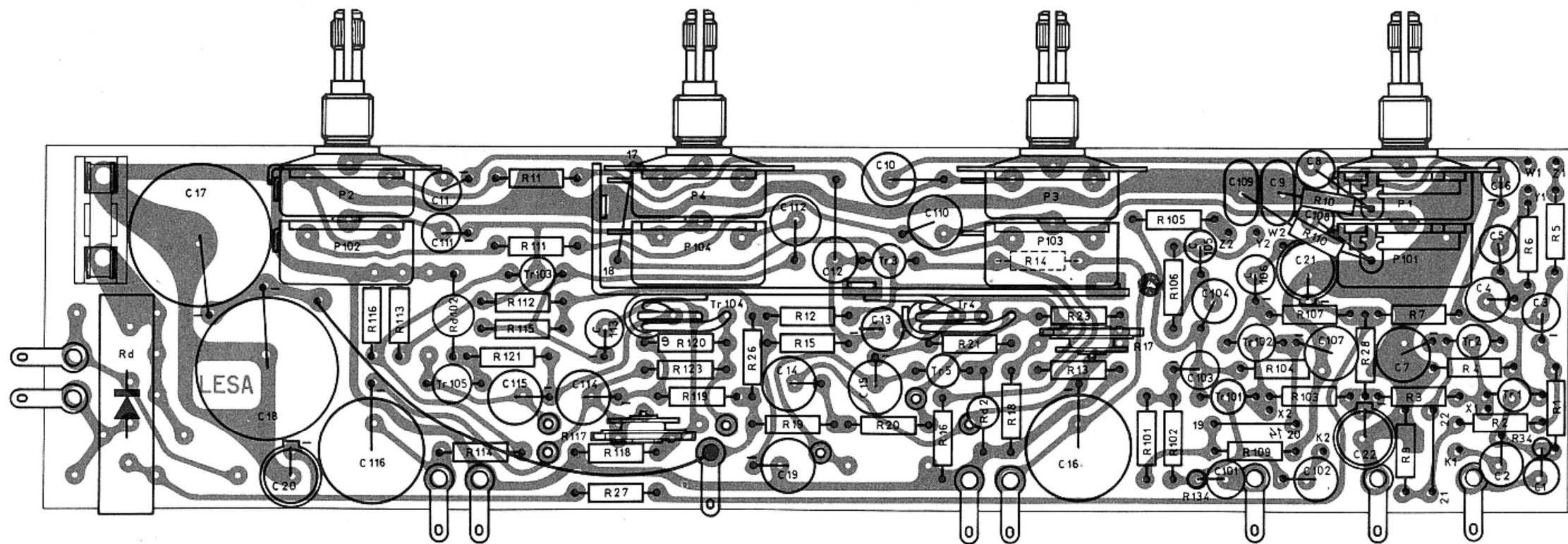
Circuito stampato - Vista lato elementi
